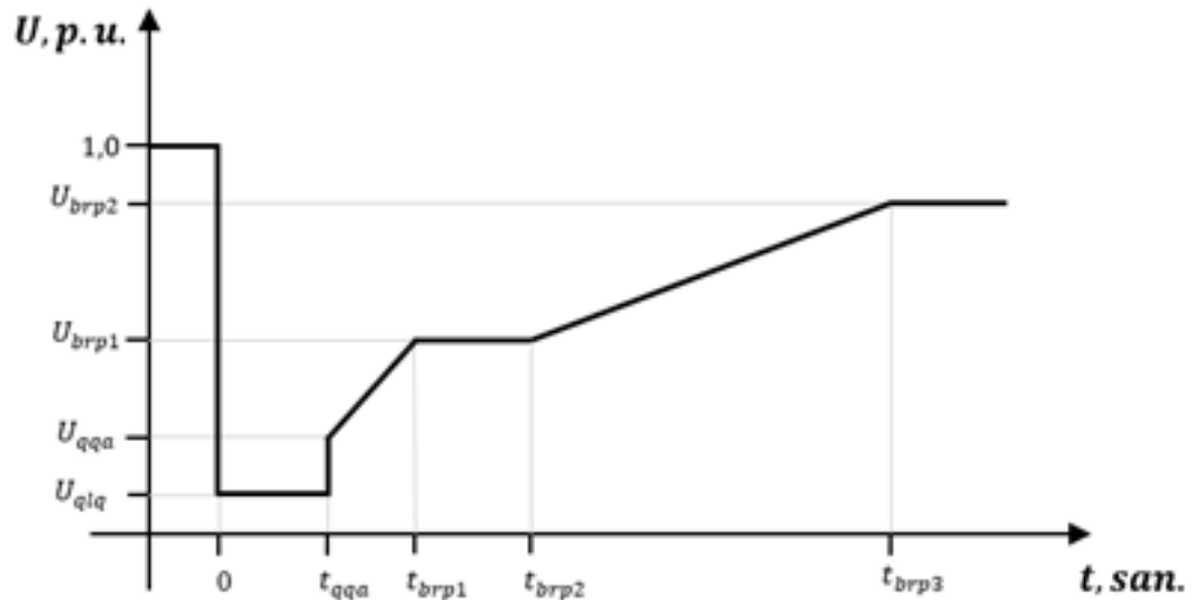
Şəkil 3. GGM-in şəbəkə qəzalarına davamlılıq profili
