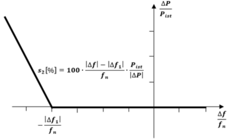
Şəkil 6. ATMHR-də GGM-in aktiv gücünün tezlik xarakteristikası
