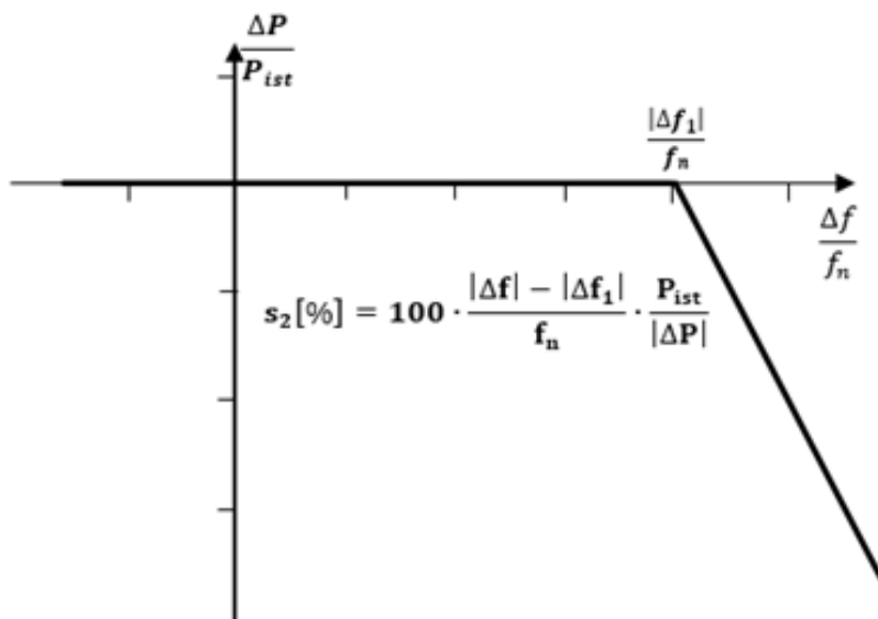
Şəkil 1. YTMHR rejimində GGM-in aktiv gücünün tezlik xarakteristikası
