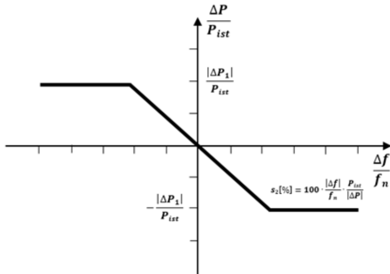
Şəkil 7. THR zamanı “ölü” zona və qeyri-həssaslıq zonası sıfıra bərabər olduqda GGM-in aktiv gücünün tezlik xarakteristikası
