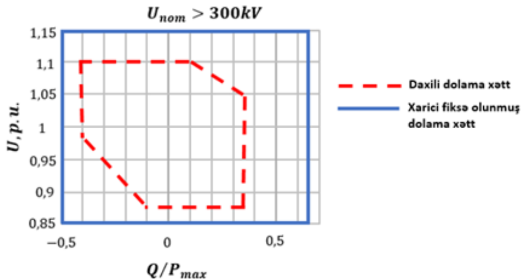
Şəkil 5. Gərginliyi 330 kV-dan aşağı olan şəbəkəyə qoşulan YGSC sistemləri üçün U \sim Q/P_{max} profili
