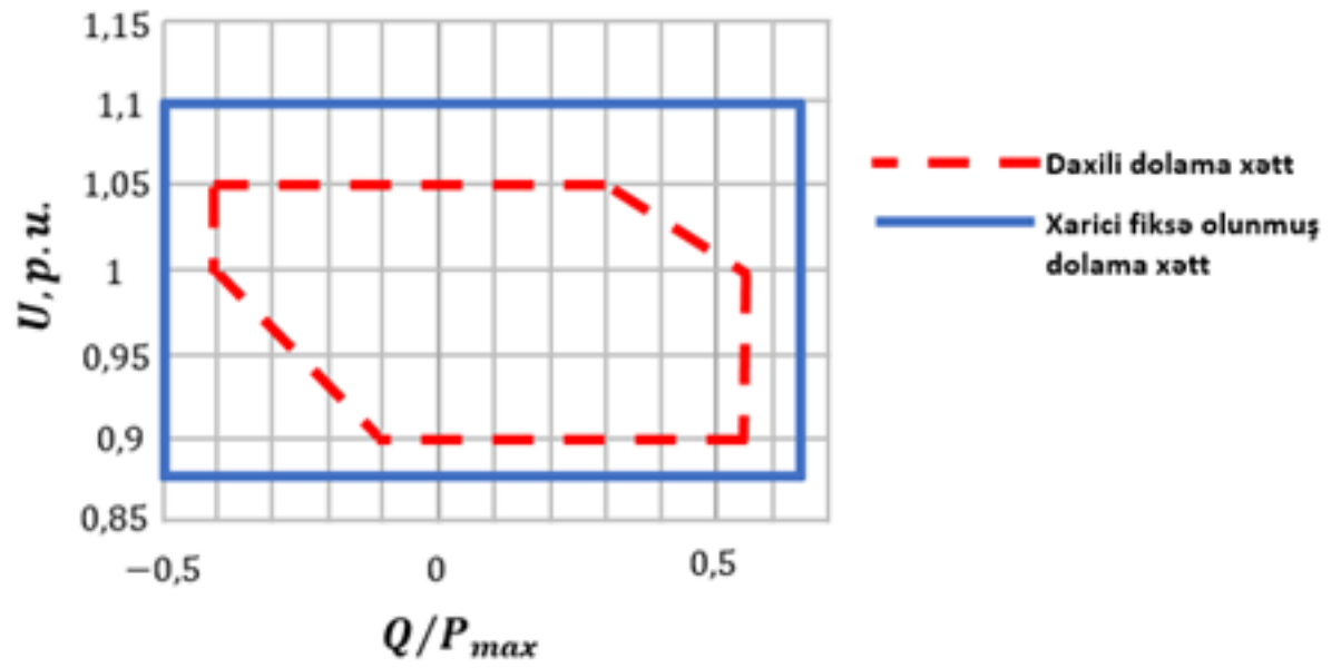
Şəkil 10. "D" tipli SGM üçün U \sim Q/P_{max} profili
