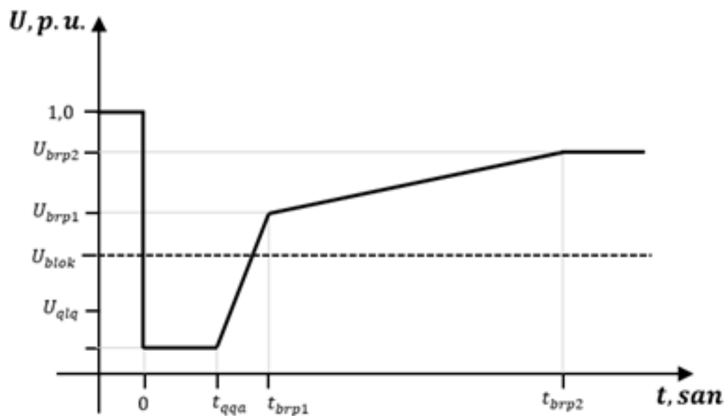
Şəkil 8. YGSC çevirici yarımstansiyasının şəbəkə qəzalarına davamlılıq (qərginlik-zaman asılılığı) xarakteristikası
